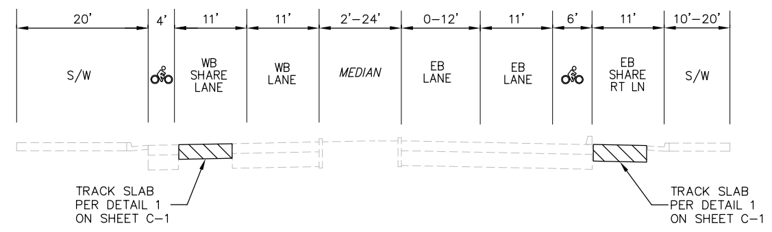
STA R 46+00 TO STA R 51+00 TOWER GATEWAY NTS
